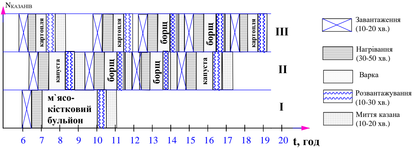
Графік роботи стаціонарних казанів для варки їжі
