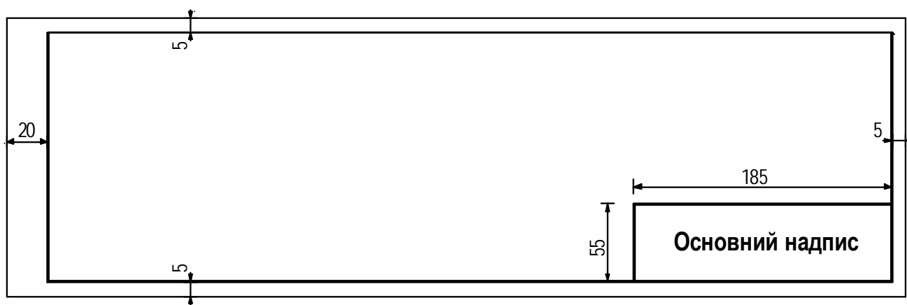
Рисунок 4.1 – Оформлення поля креслення
