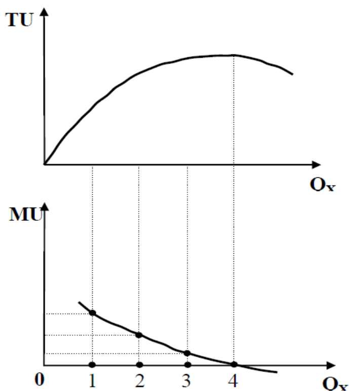
Рис. 2.1 – Зміна сукупної та граничної корисності блага X у процесі його пропорційного споживання
