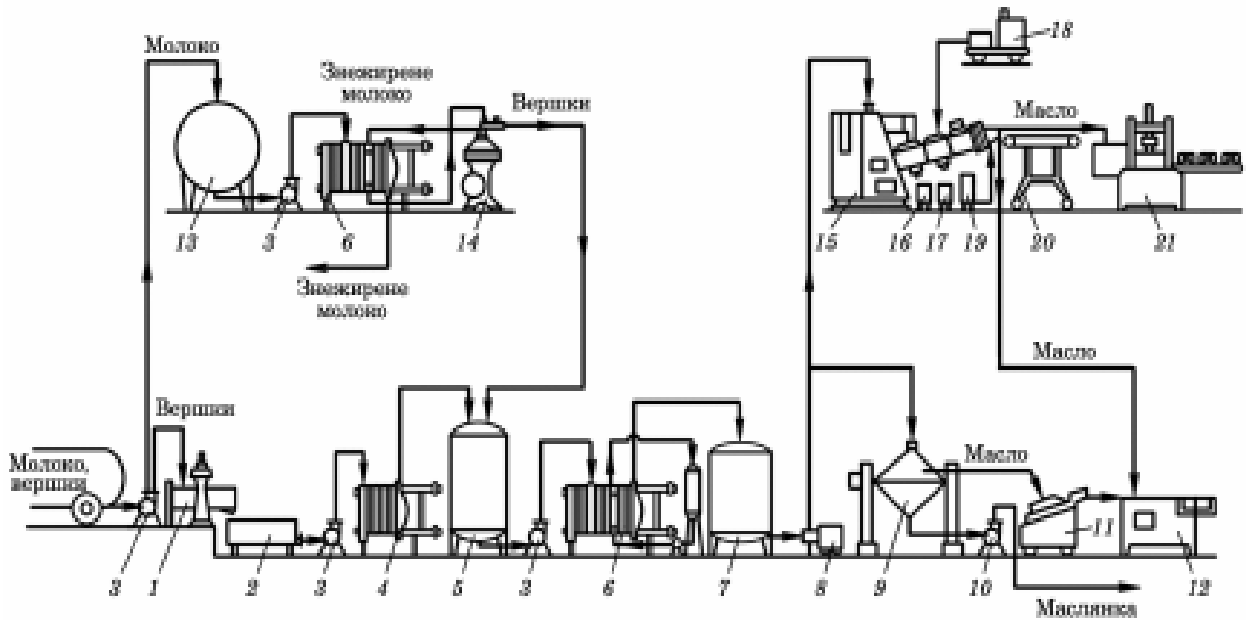
Рис. 3.17 – Апаратурна схема виробництва масла методом збивання вершків: 1 – ваги; 2 – приймальна ванна; 3 – насос; 4 – пластинчастий теплообмінник; 5 – місткість для вершків; 6 – пластинчаста пастеризаційно-оходжувальна установка з дезодоратором; 7 – місткість для визрівання вершків; 8 – гвинтовий насос; 9 – маслоготовлювач періодичної дії; 10 – насос для маслянки; 11 – гомогенізатор-пластифікатор; 12 – машина для фасування масла в коробки; 13 – місткість для молока; 14 – сепаратор-вершковідокремлювач; 15 – маслоготовлювач безперервної дії; 16 – бачок для маслянки; 17 – бачок для промивної води; 18 – пристрій для соління масла; 19 – пристрій для дозування води в масло; 20 – конвеєр для масла; 21 – автомат для дрібного фасування
