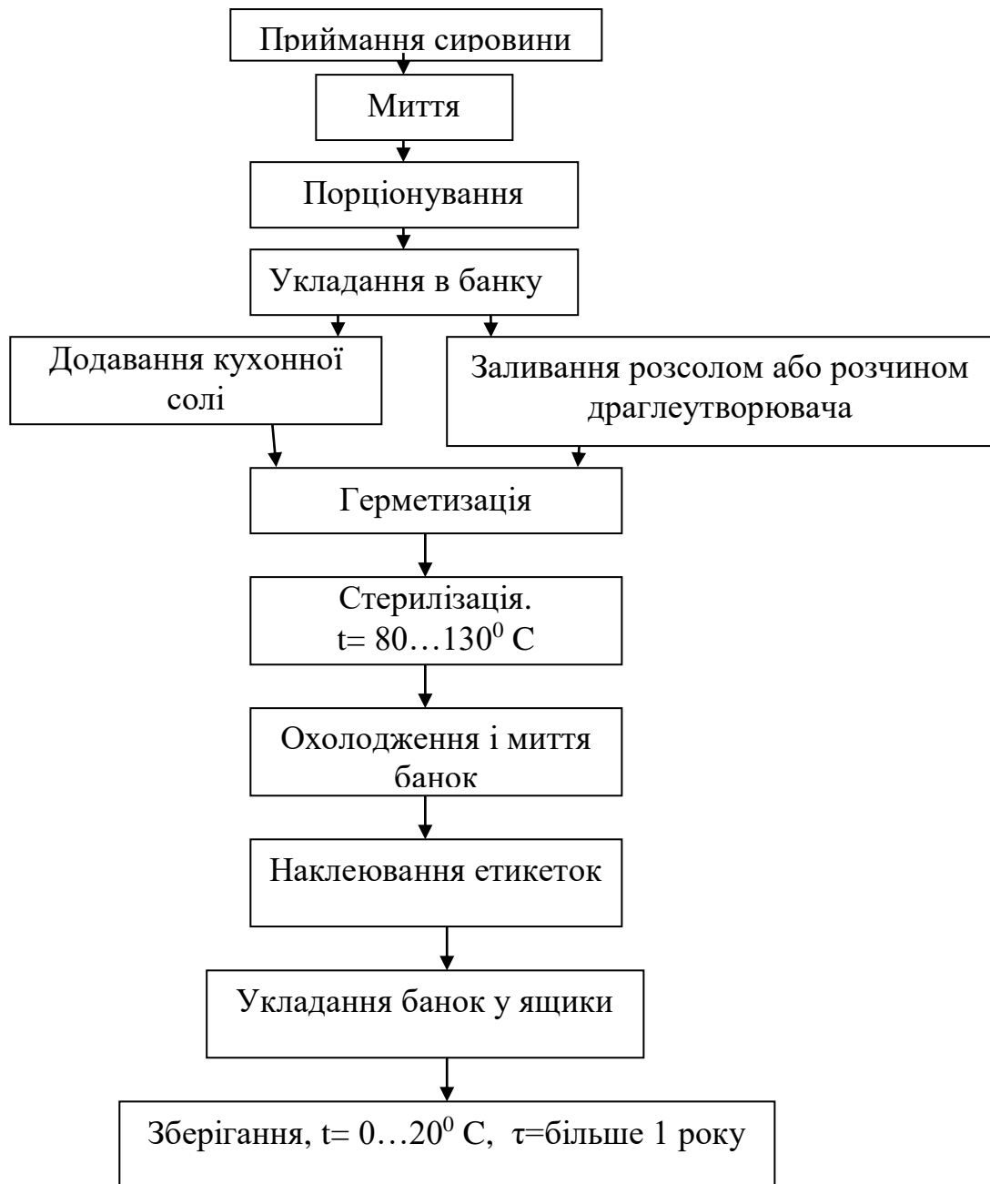
Рис. 2.17 – Технологічна схема виробництва натуральних консервів
