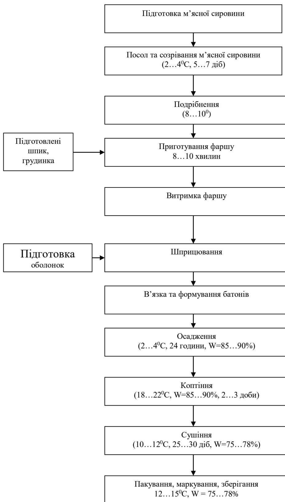
Рис. 1.48 – Технологічна схема приготування сирокопчених ковбас
