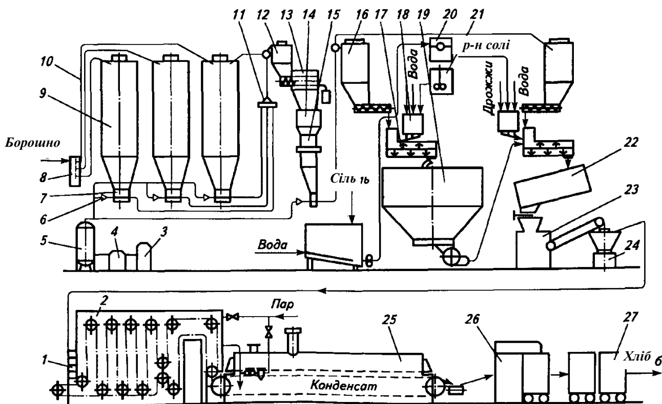
Рисунок 5.8 - Машинно-апаратна схема лінії виробництва подового хліба
