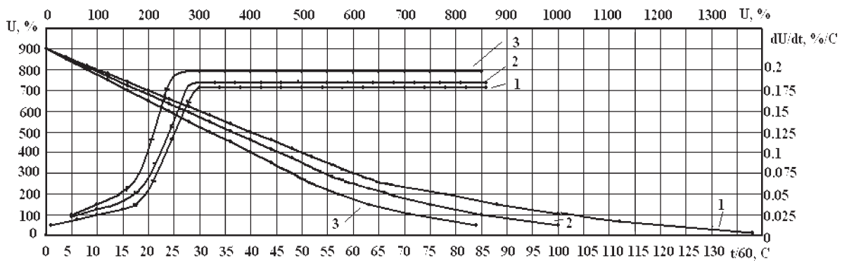
Рисунок 1 — Криві сушіння (1, 2, 3) і швидкості сушіння (1', 2', 3') печериці двоспорової в нерухомому шарі:
