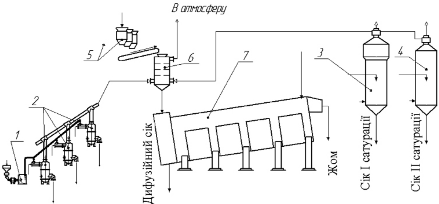
Рис. 1. Принципова схема ошпарювання бурякової стружки: 1- сиркоспалювальна піч; 2- апарати сульфитації; 3- апарат I сатурації; 4- апарат II сатурації; 5- бурякорізки; 6- ошпарювач бурякової стружки; 7- дифузійний апарат
