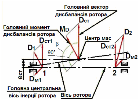
Рис. 2. Умови навантаження опор робочого органу СГМ під впливом експлуатаційних факторів [14]
