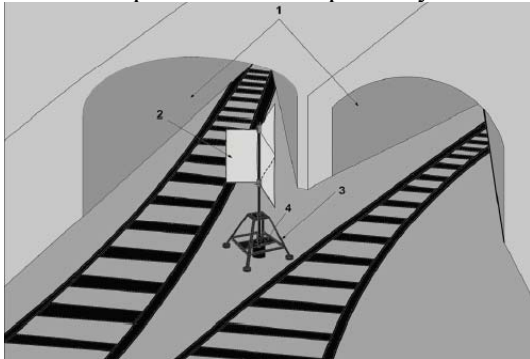
Рис. 1. Схема розташування мінівітрової електростанції у шахті: 1 – перший та другий квершлагів; 2 – лопаті вітроколеса; 3 – металева опора вітроколеса; 4 – генератор
