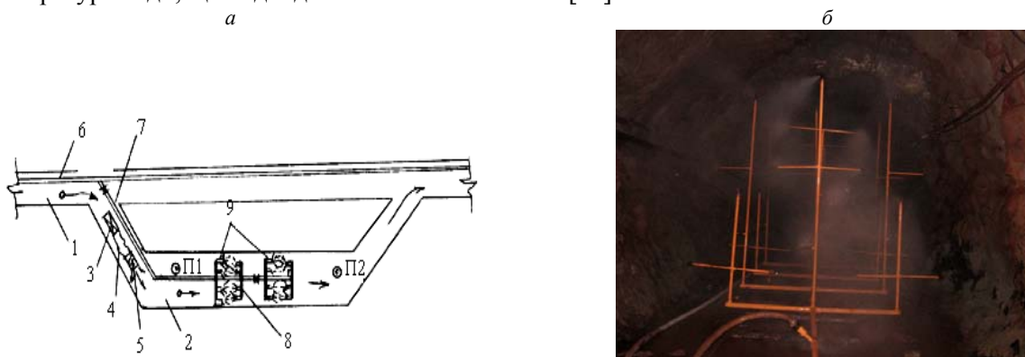
Рис. 5. Схema установки «Оазис» для проведення досліджень водо-форсункового охолодження рудникового повітря у камері зрошення: а: 1 - основна виробка; 2 - камера зрошення; 3 - вентилятор; 4 - рукав; 5 - дифузор-нагрівач; 6 - основний водопровід; 7 - магістральний водопровід; 8 - установка «Оазис»; 9 - форсунки; б - вид установки «Оазис» у камері зрошення; 10 - конденсатор
